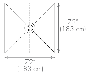
STC-TRAY183/183
