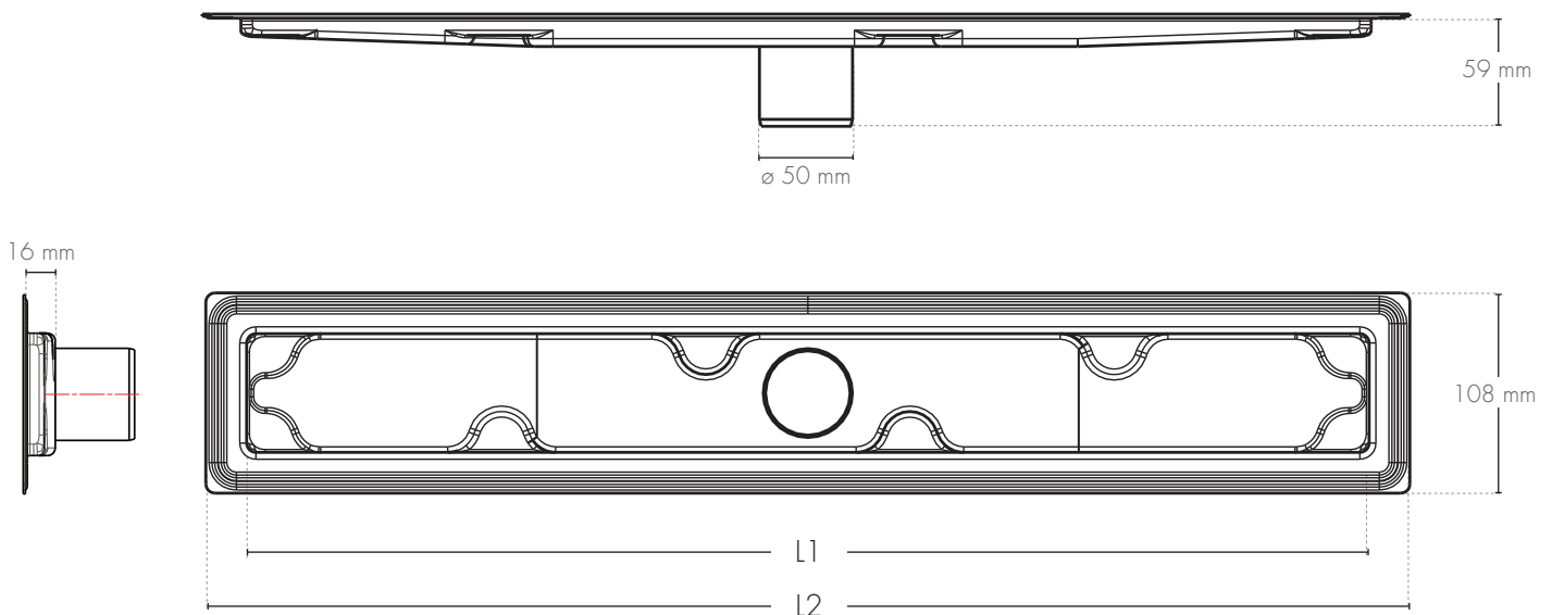
STL-BV, vertikale Abflusssrinne
