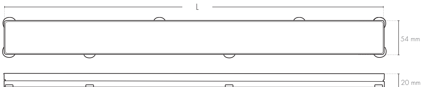
STL-CTF, cover carrelable avec bac de rétention
