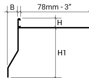
Alluminio BBS
