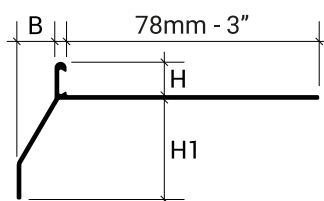
Alluminio BBS30
