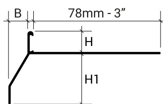
Alluminio BCS30
