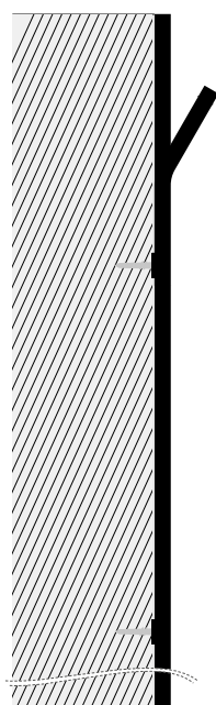
Supports de montage (100 - 835 - 830 - 835 - 100) (mm)
