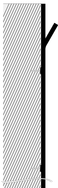
Staffe di fissaggio dall'alto (100 - 835 - 830 - 835 - 100) (mm)
