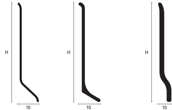
Abschnitt Edelstahl poliert Abschnitt Aluminium Abschnitt geschäumter Kunststoff
