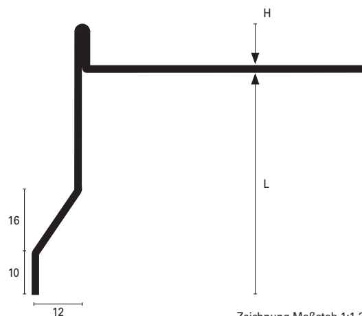
Zeichnung Maßstab 1:1,2 (BBS 55 A*)
