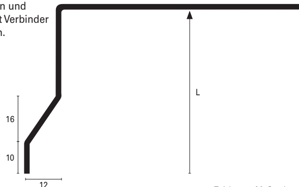
Zeichnung Maßstab 1:1 (BOS 42*)
