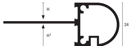
Zeichnung Maßstab 1:1 (BR 100*)
