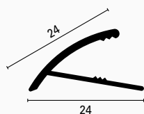
Sezione quotata scala 1:1
