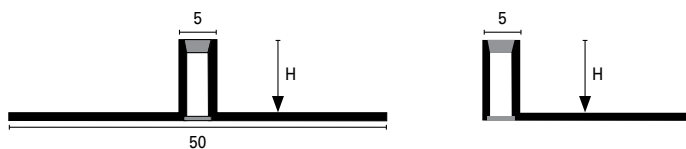
Sezione quotata scala 1:1 (CAJ 100*)
