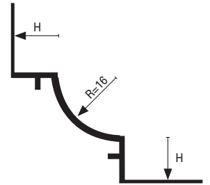
Zeichnung Maßstab 1:1
