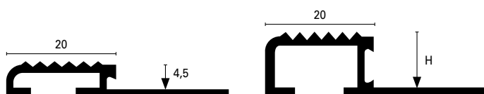
Sezione quotata scala 1:1 (FO 45* - FO 100*)
