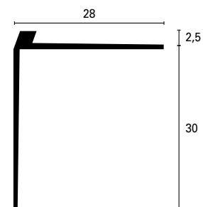
Sezione quotata scala 1:1
