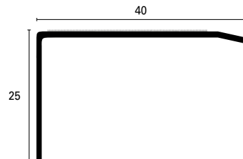
Echelle section cotée 1:1
