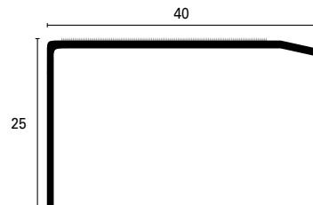
Sezione quotata scala 1:1
